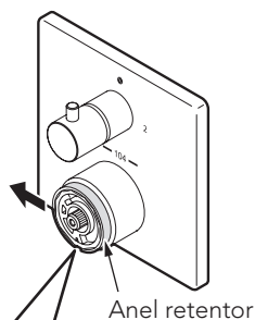
Cartucho de termóstato
