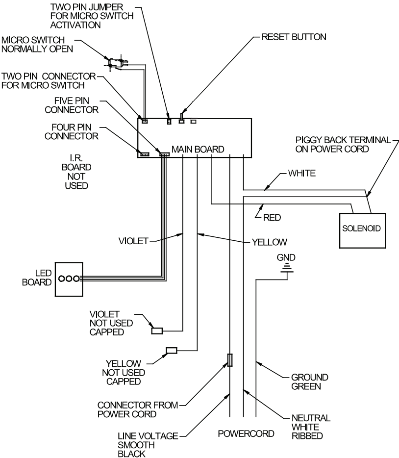
WIRING DIAGRAM 120 VOLT & 220 VOLT SINGLE & BI-LEVEL MICRO SWITCH ACTIVATION Fig. 11
