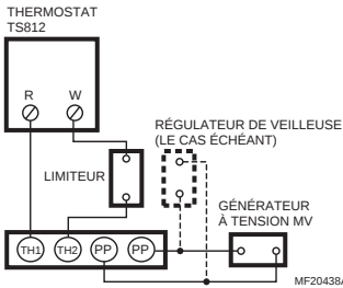
Fig. 5. Schéma de raccordement typique d'un TS812A à un système à tension mv.
