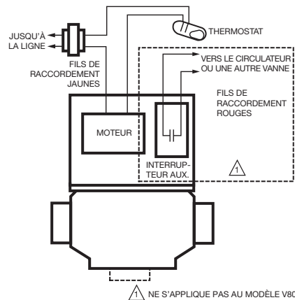
Fig. 5. Câblage typique des vannes V8043A, V8043E.
