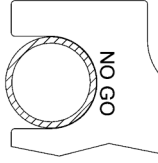
Figure 2 – Sertissages hors tolérances
