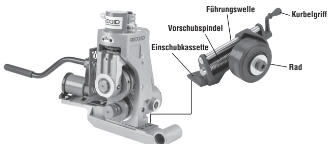
Abbildung 1 - Stabilisator am 918 Rollnutgerät
