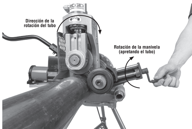
Figura 3 – Posición del estabilizador
