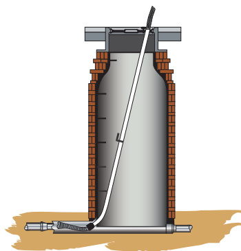
A-17 Manhole Guide Pipe
