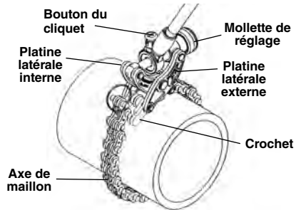
Figure 5 – Coupe-tubes à chaîne nos 206 et 246
