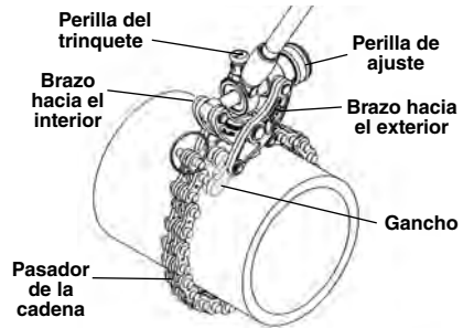
Figura 5 – Cortadora de tubos cloacales 206/246
