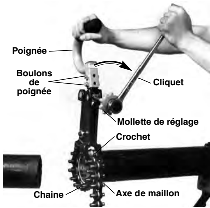
Figure 4 – Utilisation du coupe-tube à chaîne no 226
